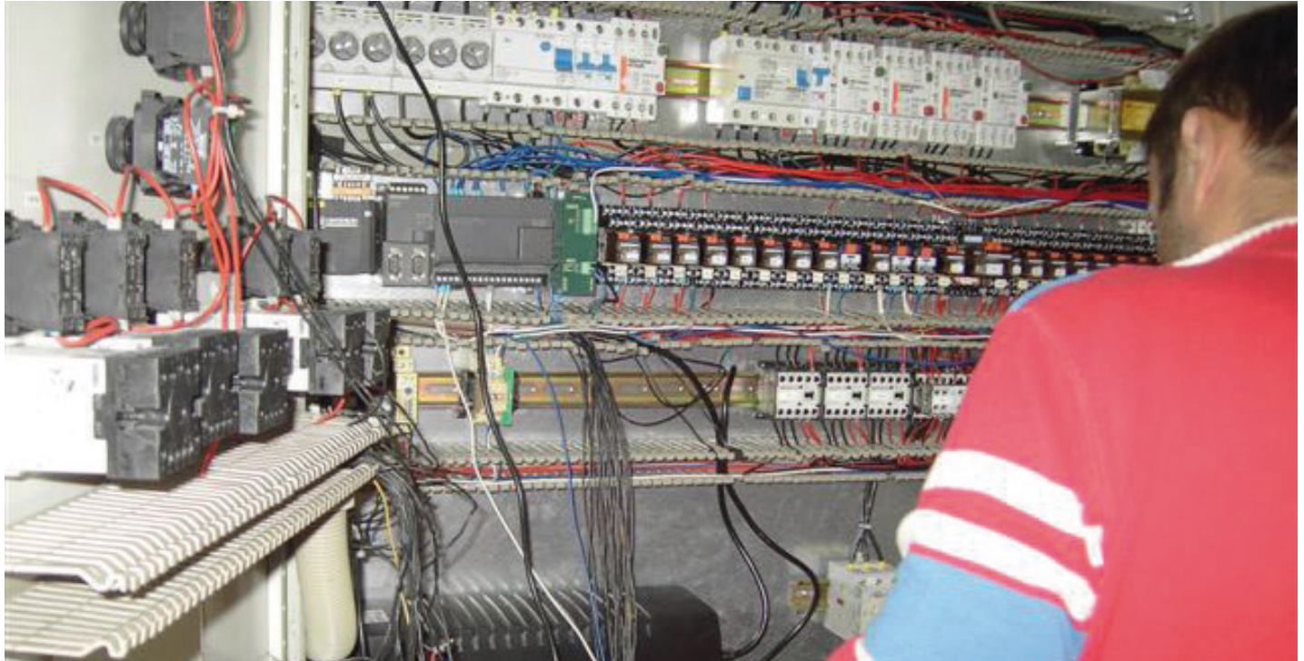
Umbau Steuerung auf SPS-Steuerung
