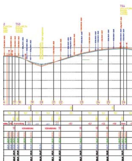
Längenschnitt
